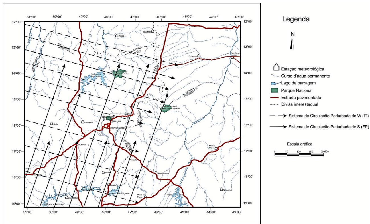
Figura 2. Sistema de circulação atmosférica perturbada em parte da Região Centro-Oeste
