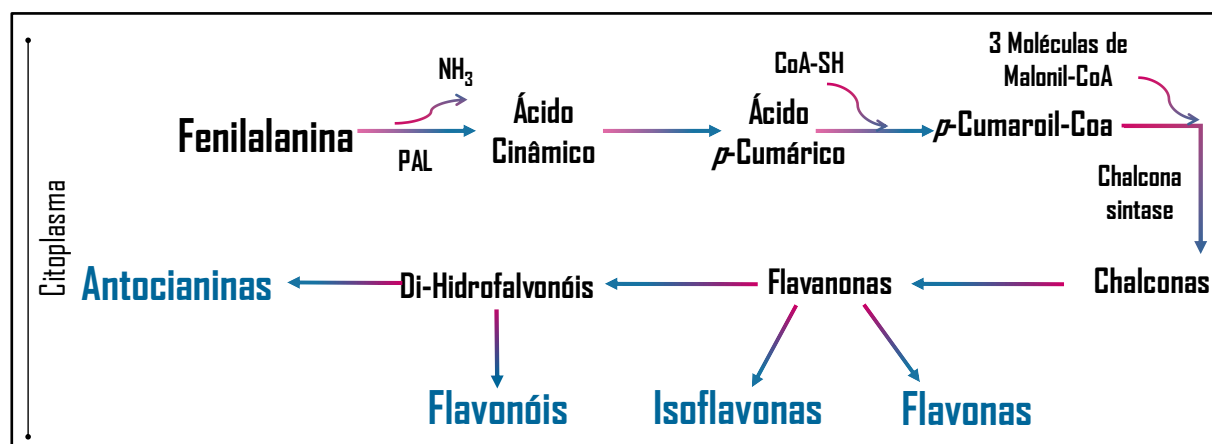
Figura 2. Fluxograma simplificado da rota de produção dos compostos fenólicos, adaptado de Taiz e Zeiger (2009).
