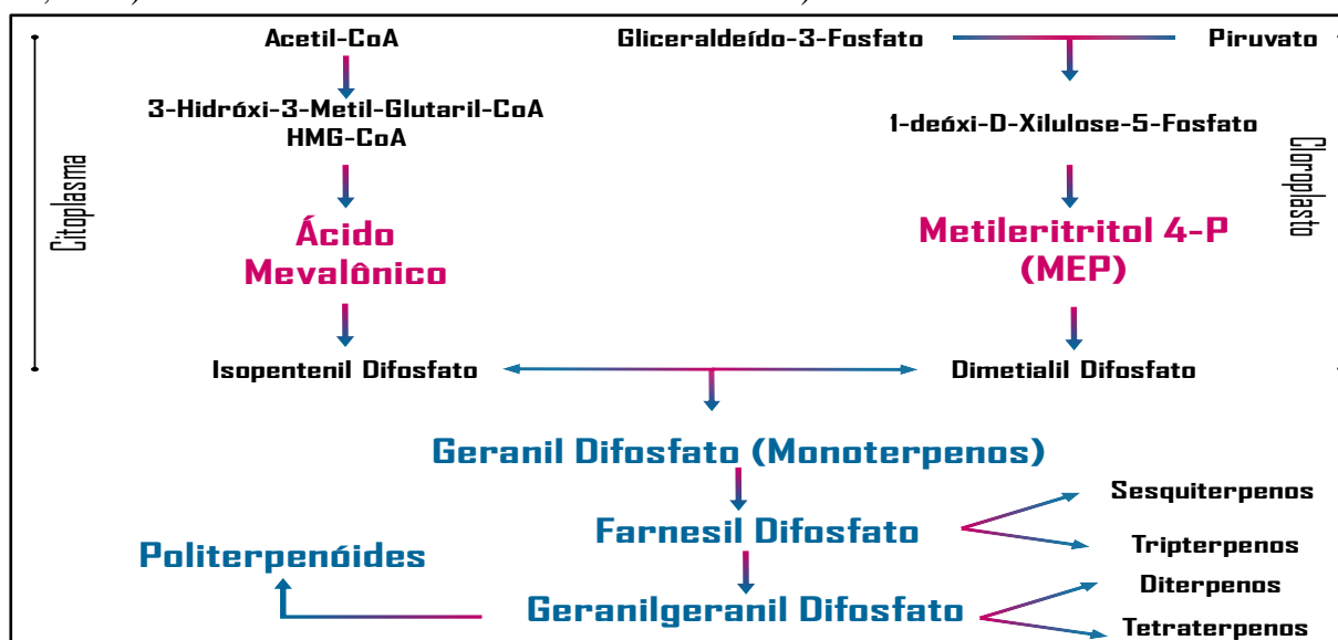
Figura 1. Fluxograma simplificado da rota de biossíntese de terpenos, adaptado de Taiz e Zeiger (2009).
