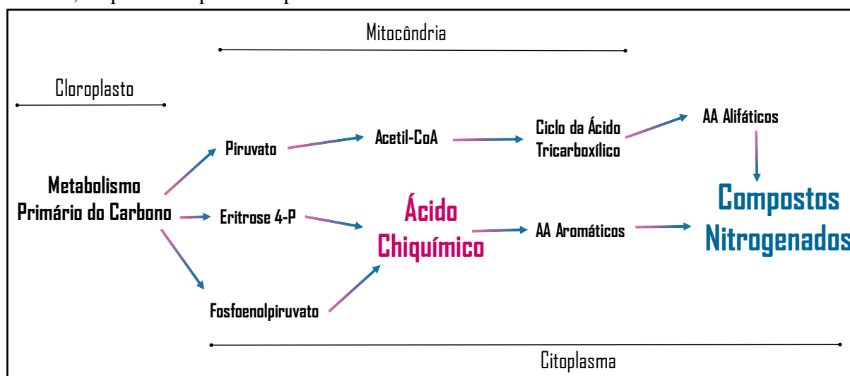
Figura 3. Rota de biossíntese de compostos nitrogenados simplificado, adaptado de Anulika et al. (2016).
